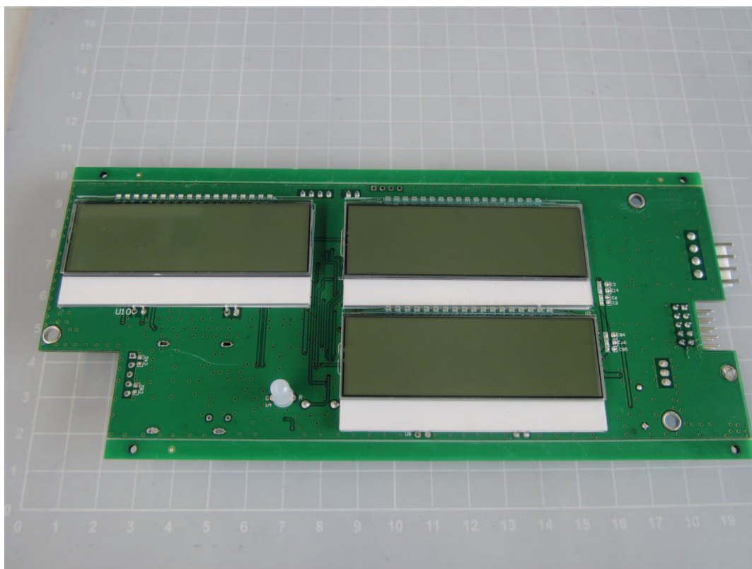
Hauptplatine, Passend für Modell KERN RFC
