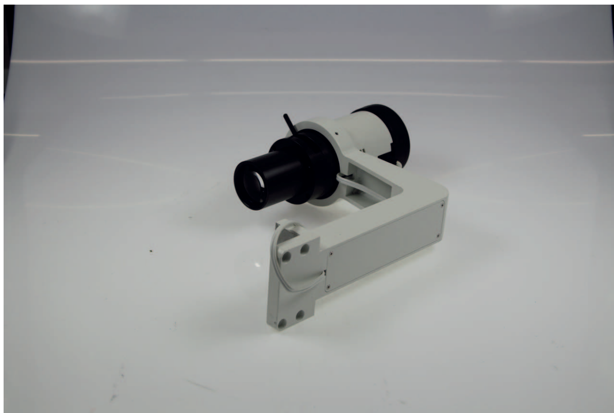
Condensador de Abbe NA (con diafragma de apertura)
