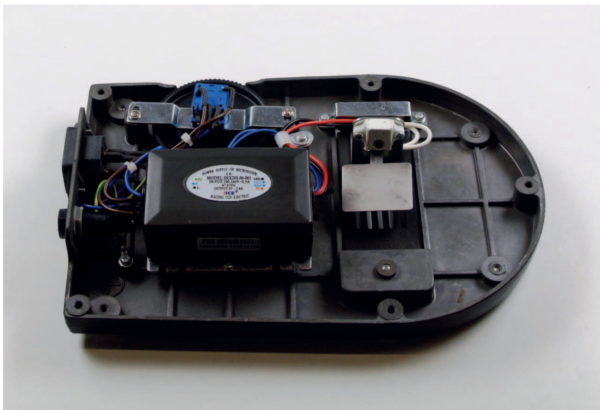
Transformator, Passend für Modell KERN OPE-1
