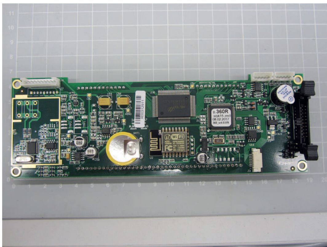
Hauptplatine RPLJ-C-2003
