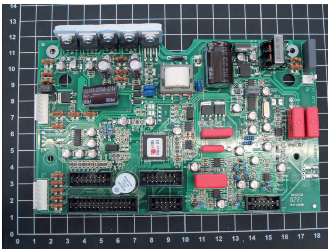
Hauptplatine, Passend für Modell KERN ALT-B
