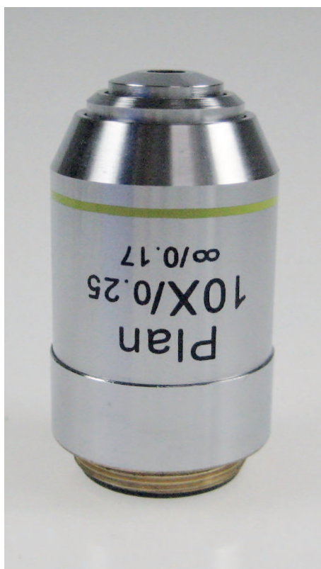
Objectif planachromatique Infinity 10 x /0,25 W.D. (4,64 mm)
