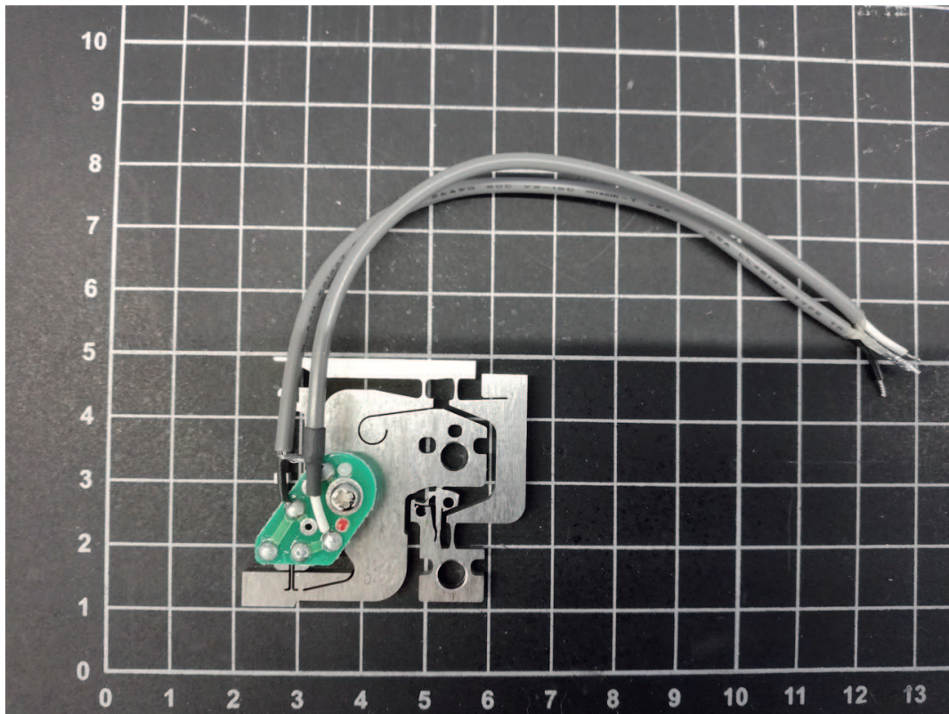
Stimmgabelfühler
