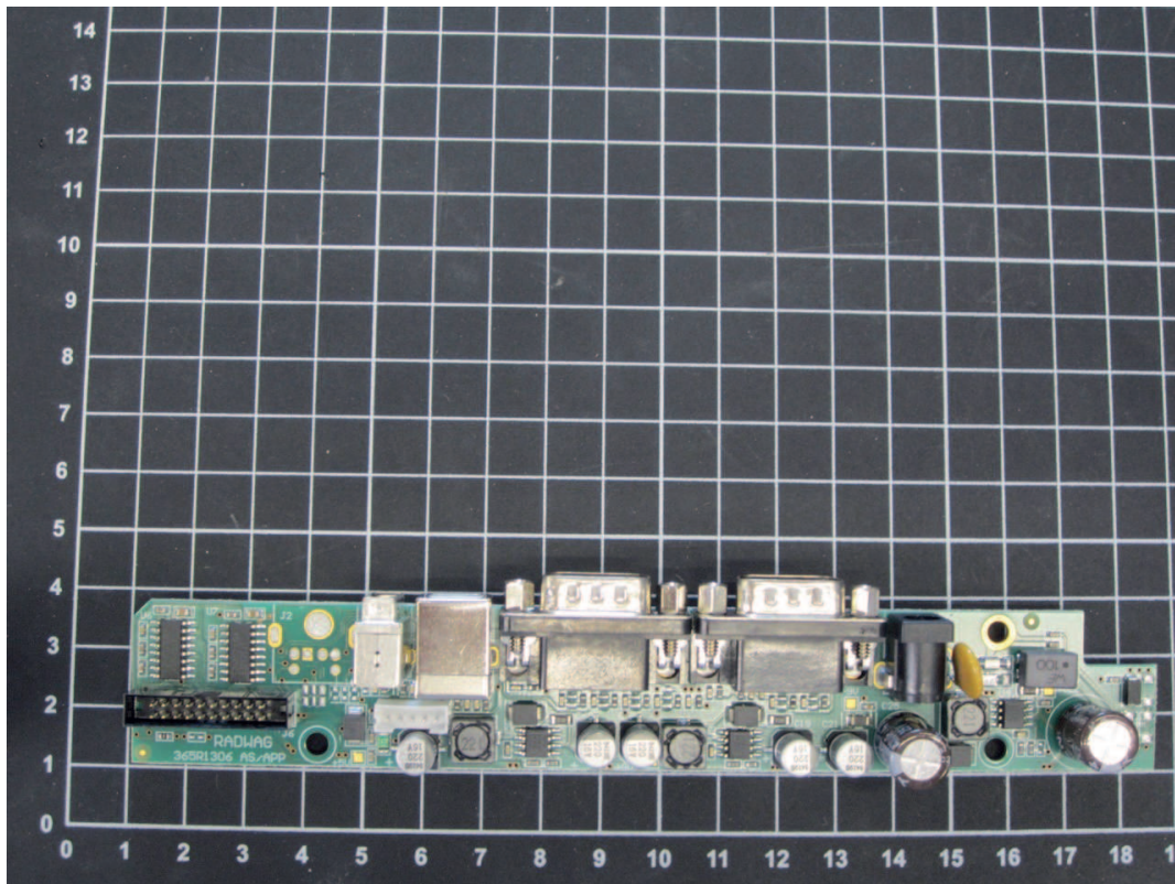
Platine, Stromversorgung, Passend für Modell KERN AEJ-C, AEJ-D
