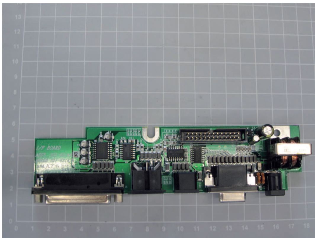
Platine, Stromversorgung
