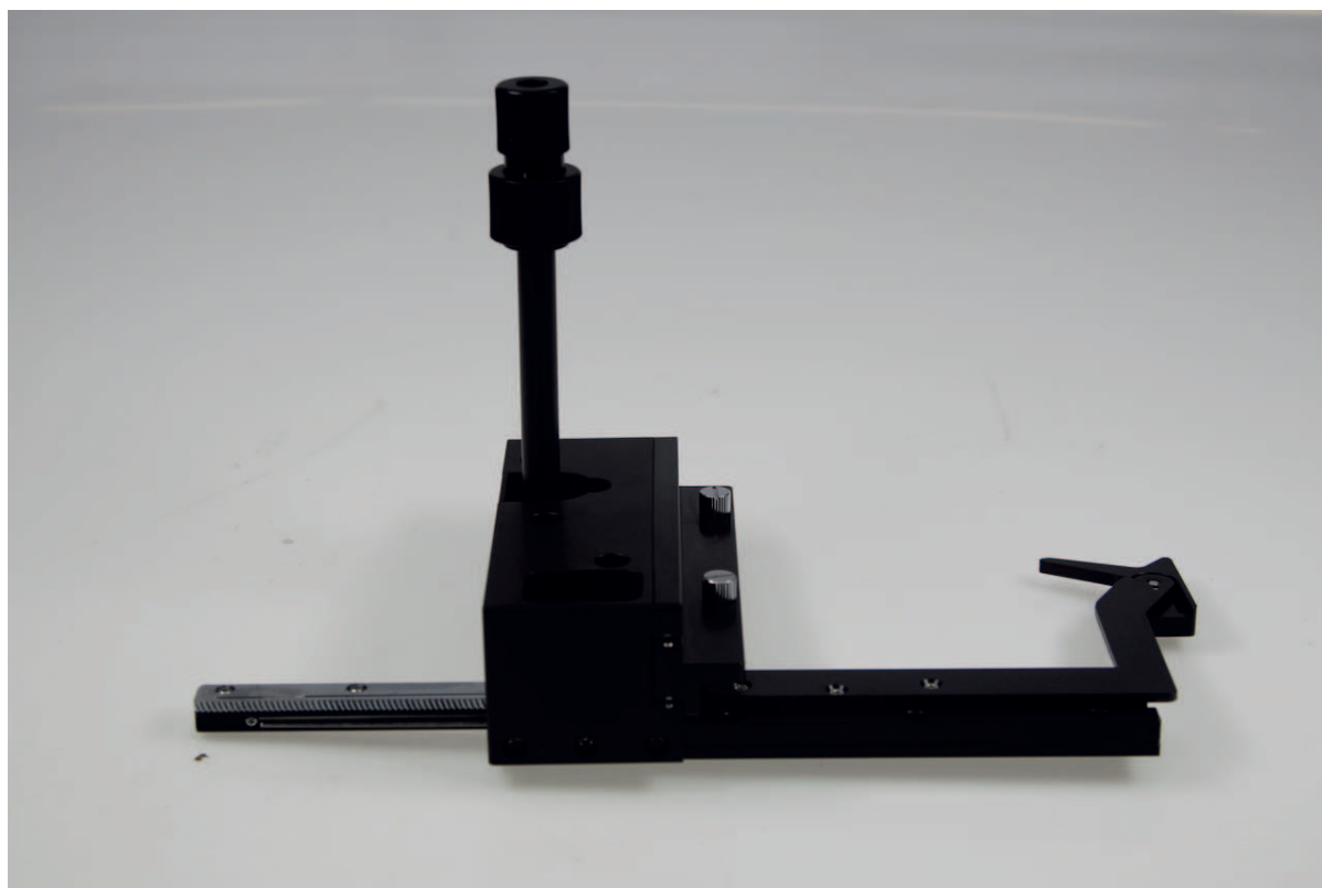
Complément mécanique de table pour microscopes inversés
