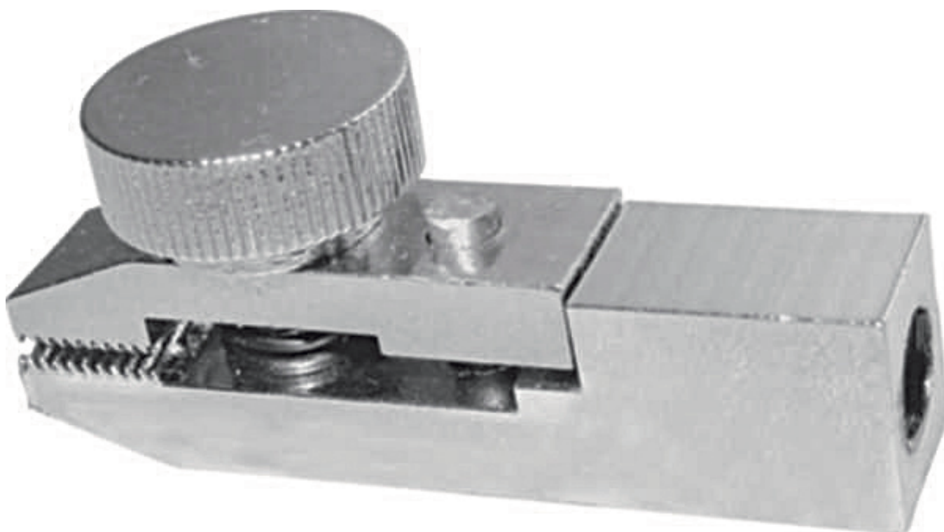
Langklammer für Zug- und Reißtests
