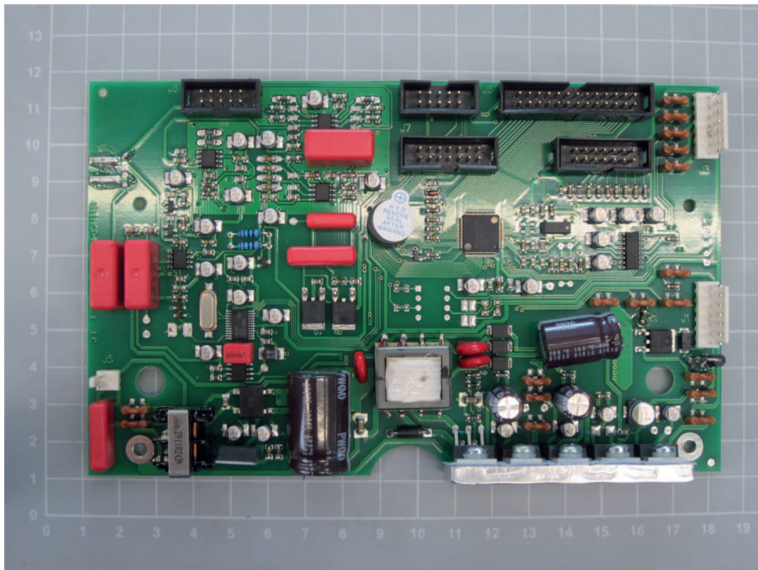
Carte mère, Convient pour le modèle KERN PLS-A, PLJ-A
