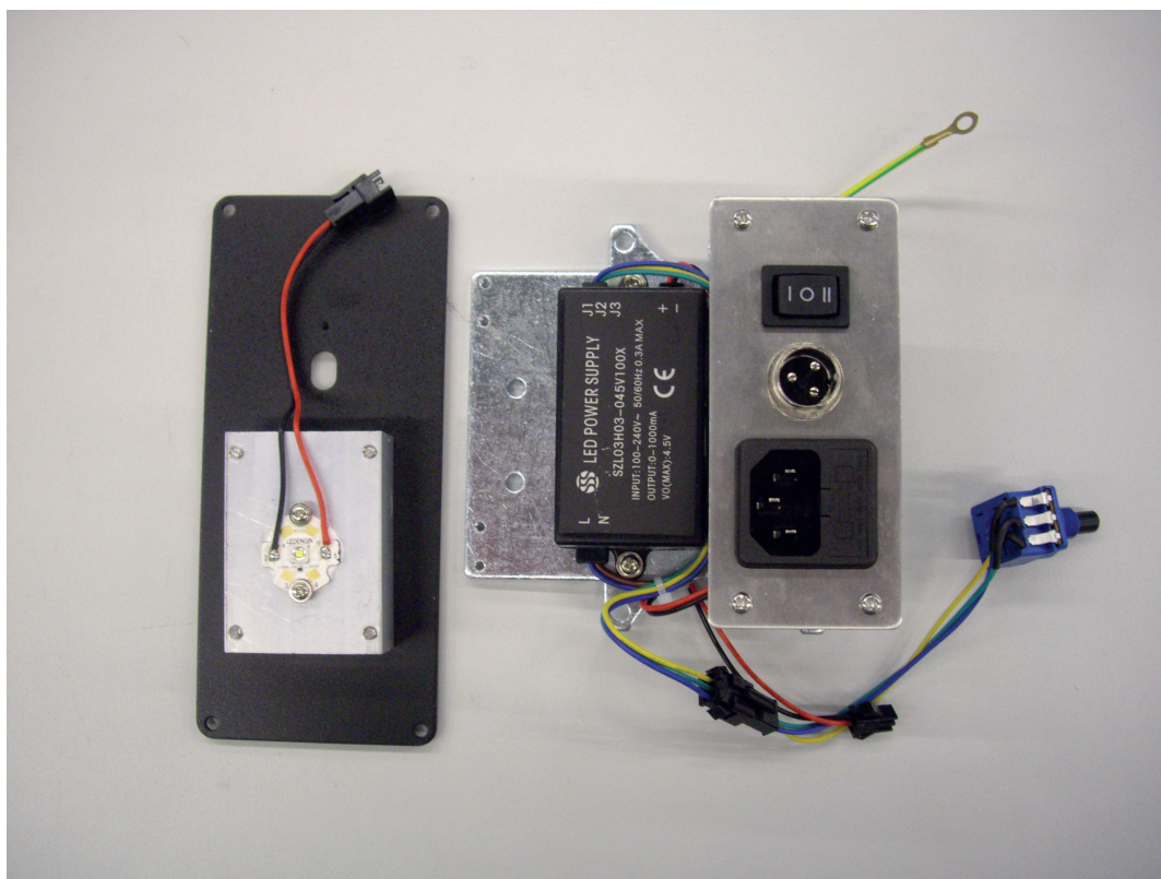
Transformateur (LED)
