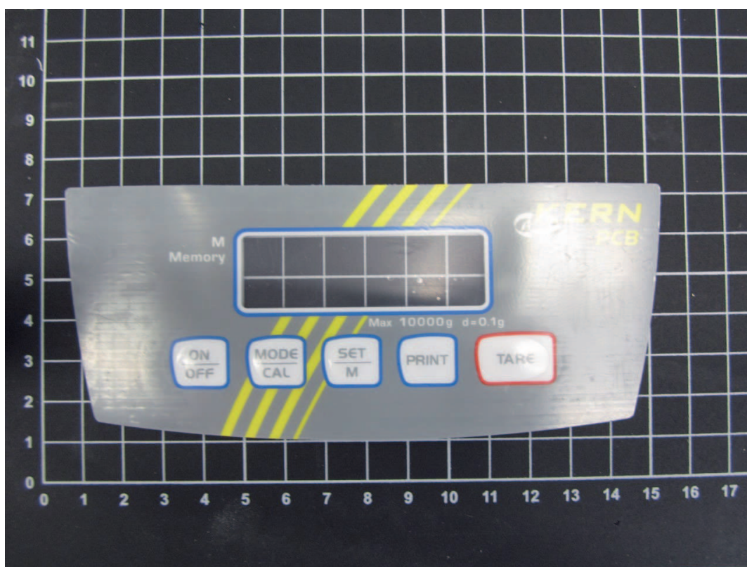
Lámina de teclado, Adecuado para modelo KERN PCB 10000-1
