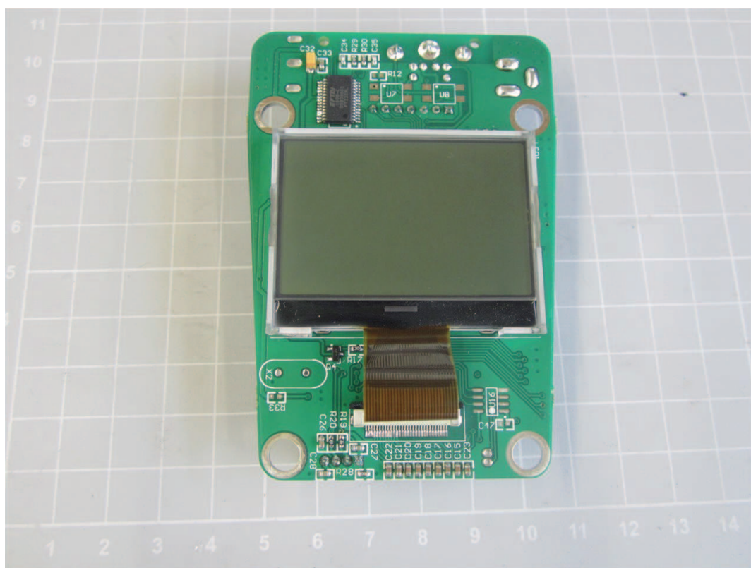
Hauptplatine RDB-2001
