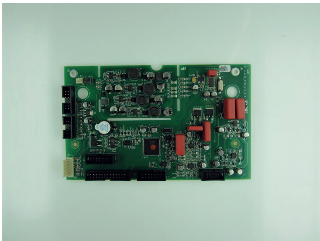
Hauptplatine RALJA-2004
