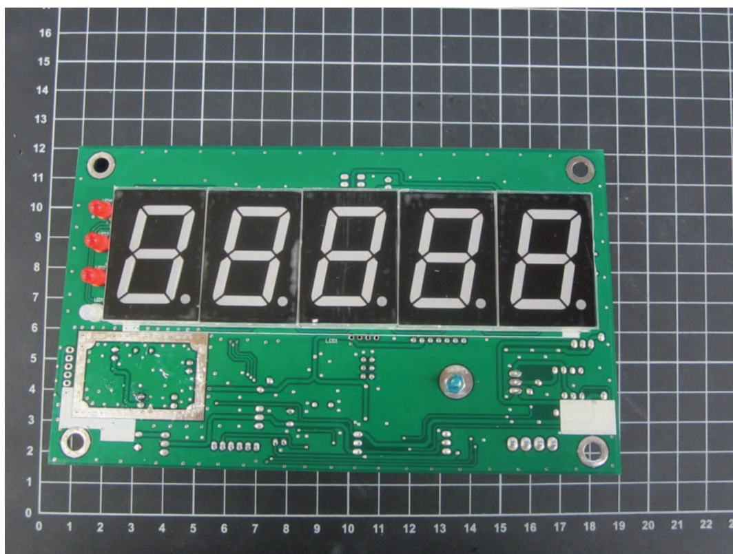
Hauptplatine, Passend für Modell KERN HFM
