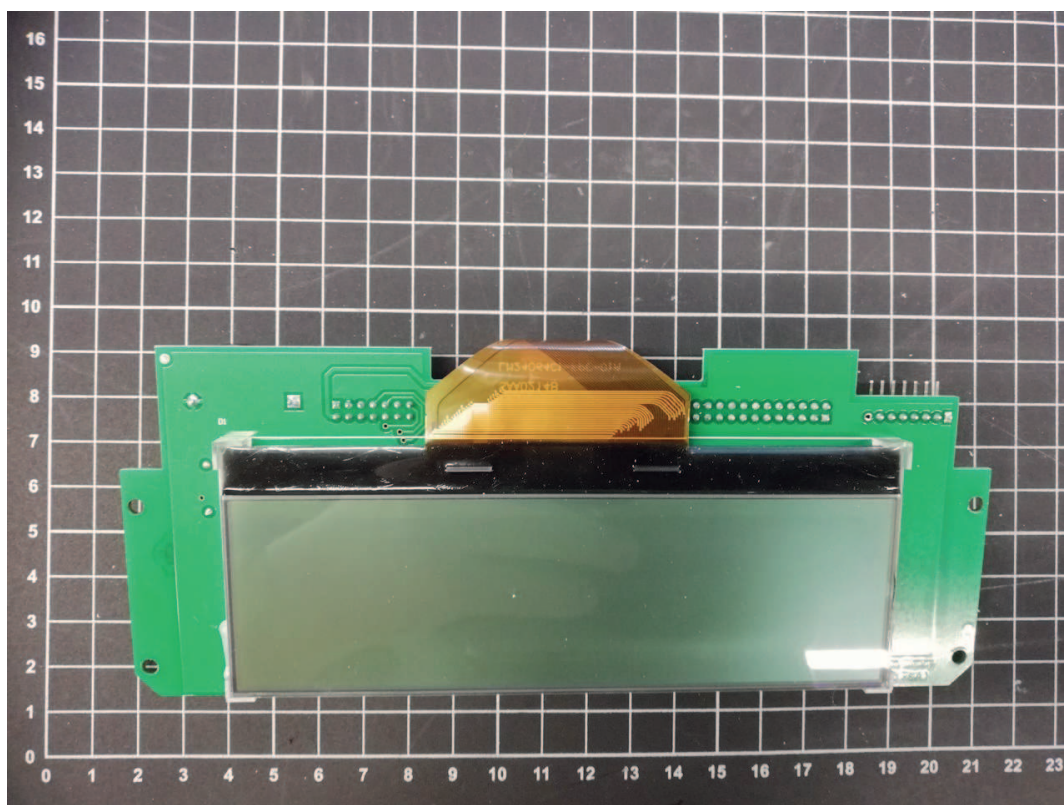
Circuito di visualizzazione
