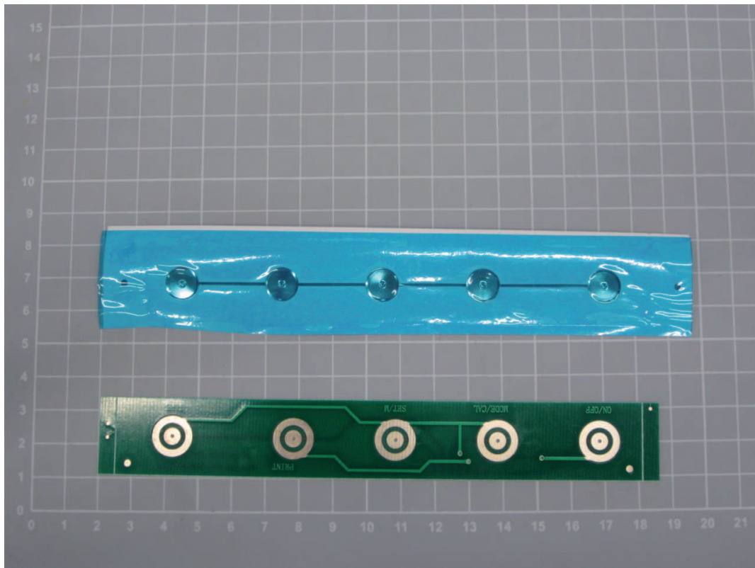
Tastaturplatine, 156x24 mm, Passend für Modell KERN DE-D, DE-A
