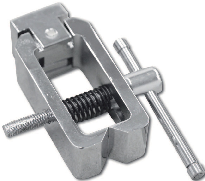
Schraubspannklemme für Zug- und Reißtests
