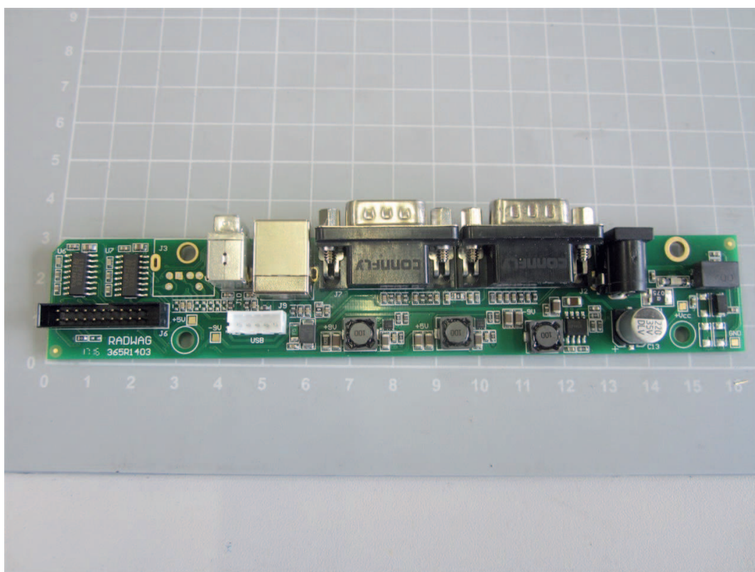
Platine, Schnittstelle
