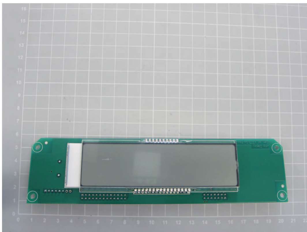
LCD Display mit Platine, Passend für Modell KERN PLS-A, PLJ-A, PLS-F, PLJ-F, ALS-A, ALJ-A
