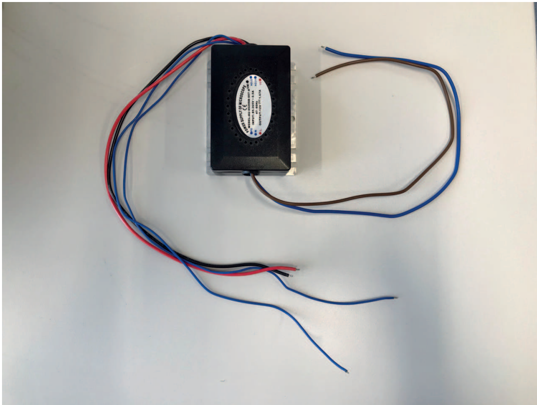
Trasformatore 12V / 20W
