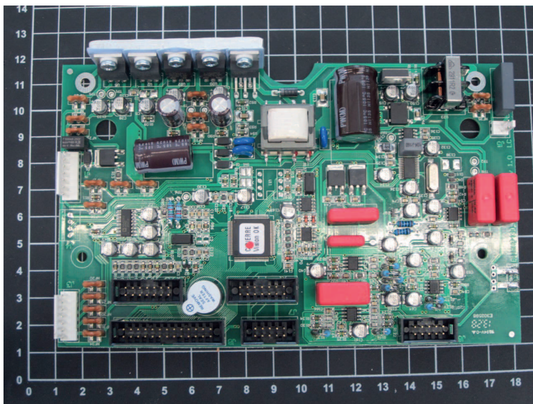
Carte mère, Convient pour le modèle KERN ALT-B
