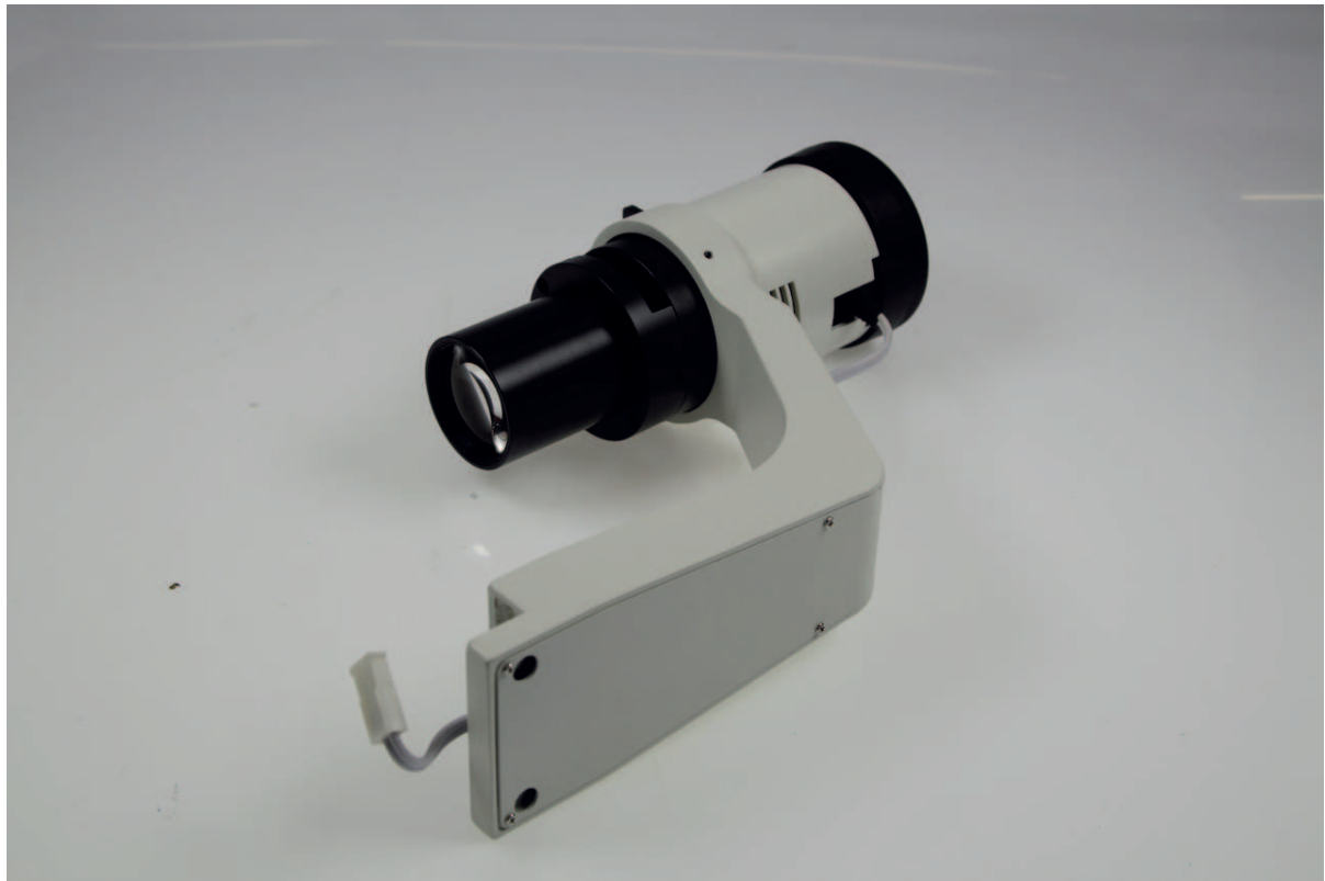
Kondensor Abbe NA (mit Aperturblende)
