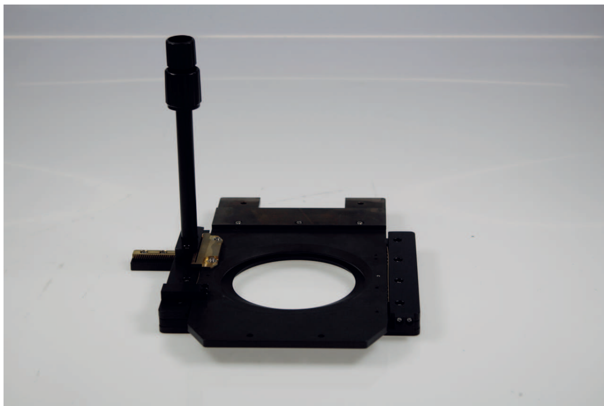
Mesa en cruz para microscopios invertidos
